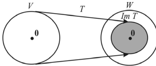
Figura 3.5: Representação gráfica da imagem de T .
