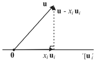
Figura 5.1: Projeção de \mathbf{u} sobre [\mathbf{u}_i] .
