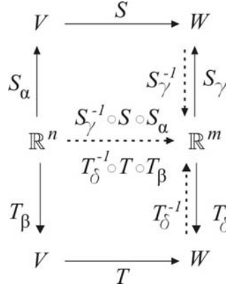
Figura 3.10: Diagrama de composição
