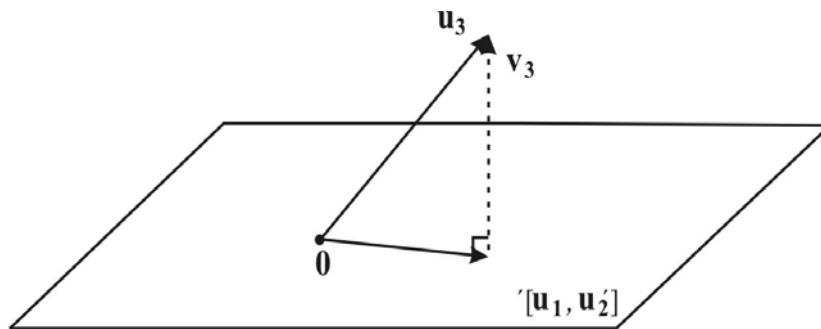
Figura 5.2: Projeção de \mathbf{u}_3 sobre o espaço [\mathbf{u}_1, \mathbf{u}_2] .
